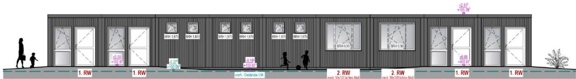
WEST ANSICHT
